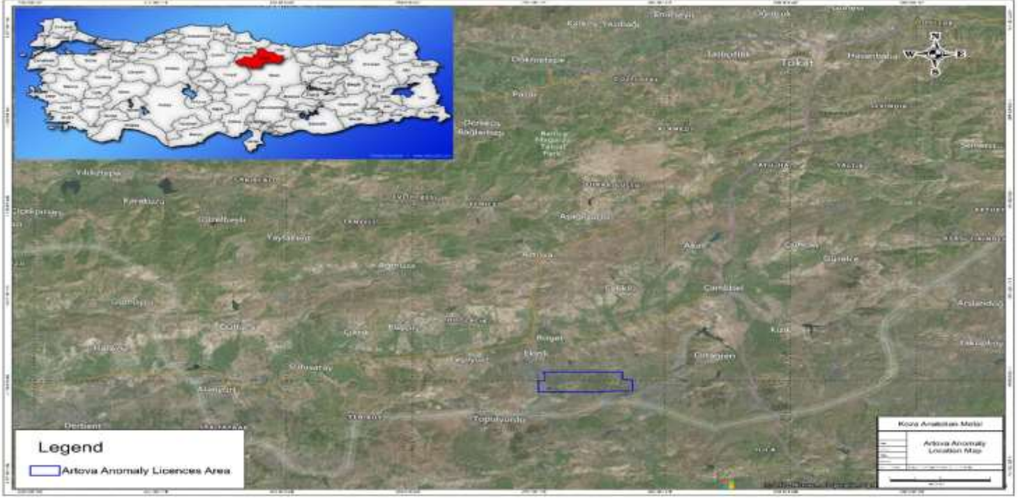
Artova Anomalisi Ruhsatlarına Ait Google Earth Uydu Görüntüsü
